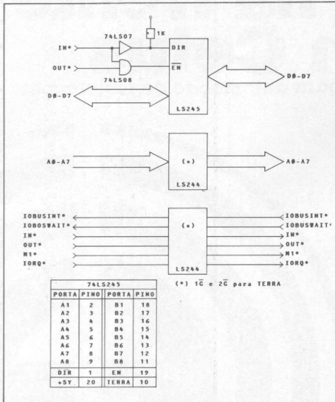
Figura 8 - Buffer para a via de E/S
